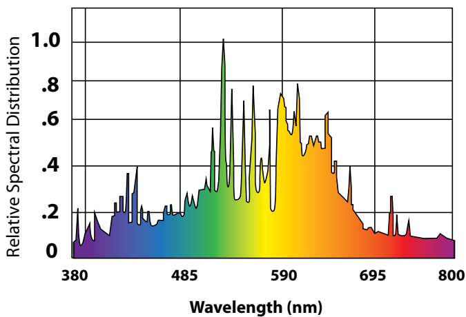
Ushio 3100K - 315W Lamp (US5002536)
